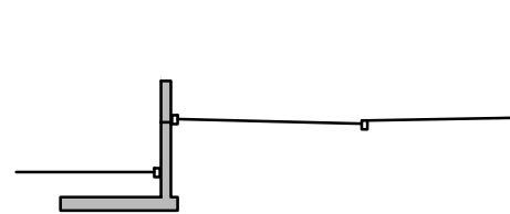
PERIAATELEIKKAUS D-D
